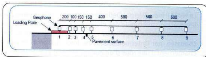
Figure 3: Schéma de positionnement des géophones.
