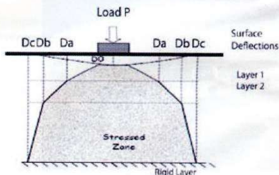
Figure 6: Analyse du bassin de déflexion de l'HWD
