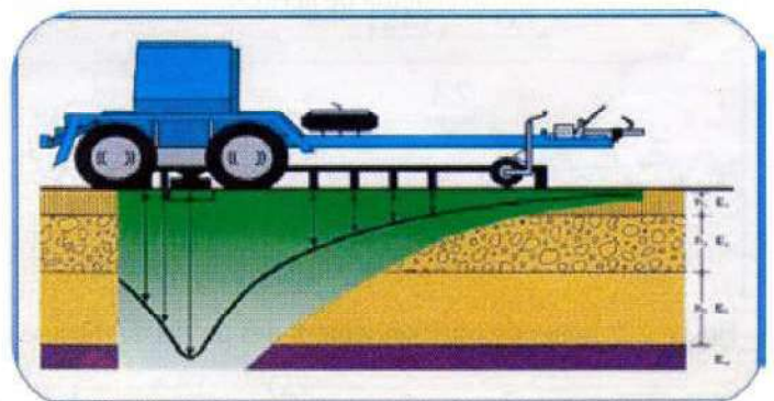
Figure 2: Schéma du principe de l'essai HWD.
