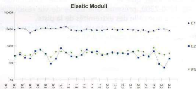
Figure 8: Module de rigidité des couches du corps de chaussée
