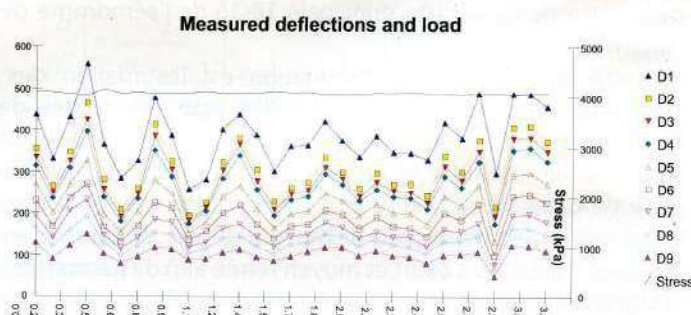
Figure 5: Déflexions de la bande axiale de la PP.
