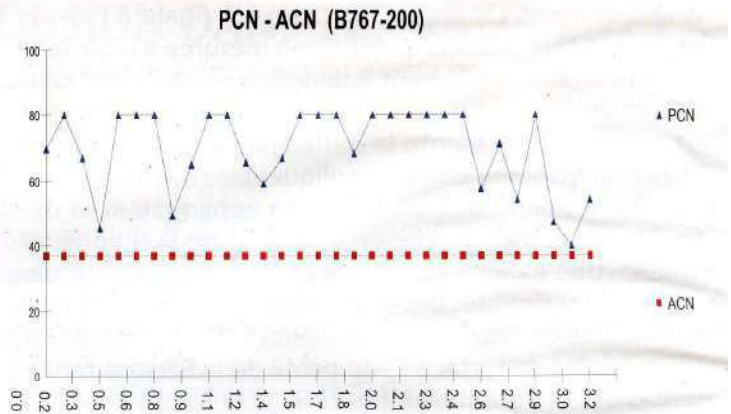
Figure 11: Valeurs de PCN de la bande axiale de la PP.
